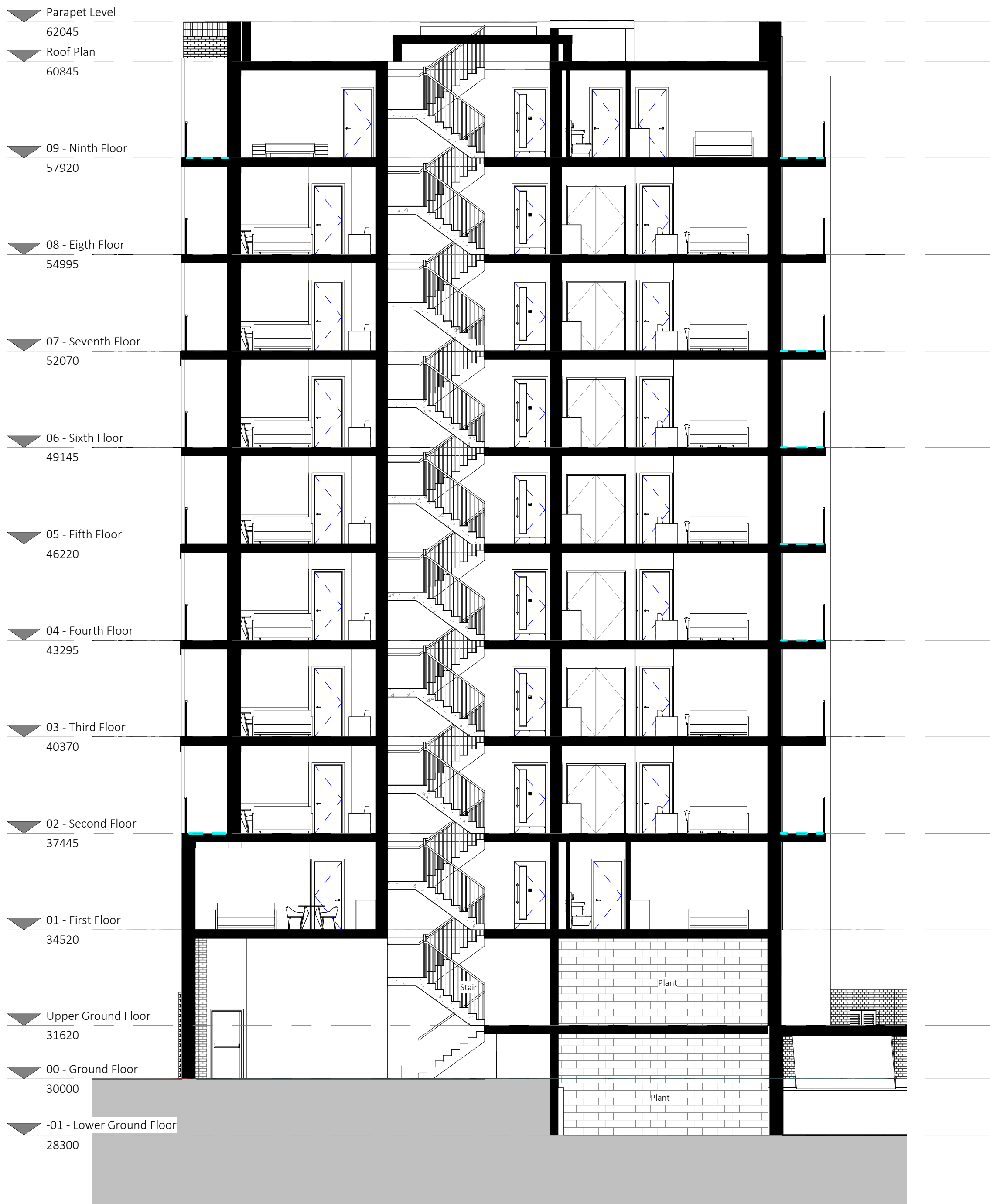
Section C-C 1 : 100
