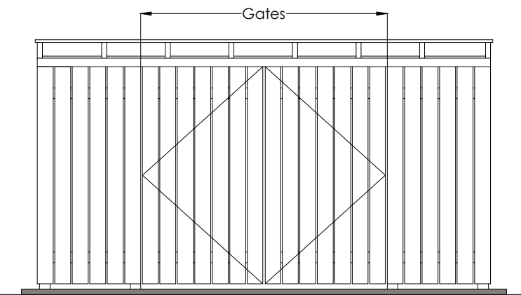
Elevation A
